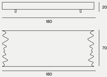
DIMENSIONS 180X70X20H
