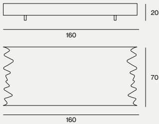
DIMENSIONS 160X70X20H
